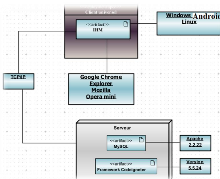
Figure 7: Diagramme de déploiement
